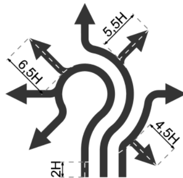
Acceso a glorieta con tres carriles.
